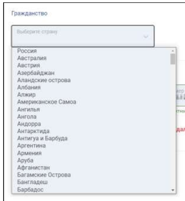
Рис. 28. Блок Гражданство
