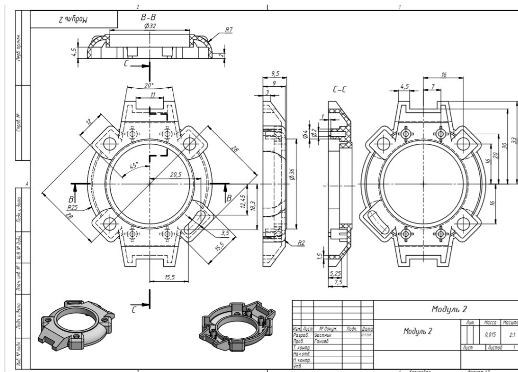
Рисунок 1 – Чертеж и 3-Д модель детали
